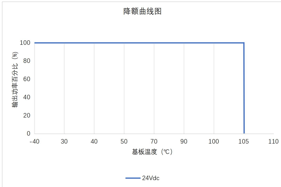
图 6.1 降额曲线图
