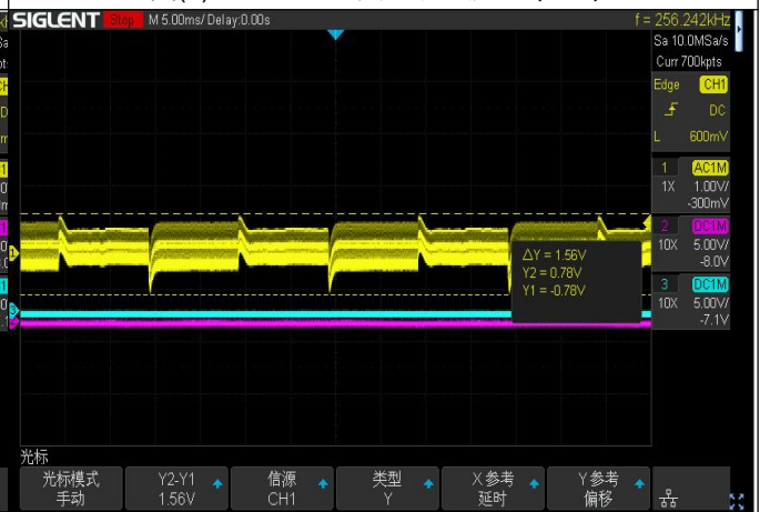
图(6) 50% ~ 75%负载动态波形 (28V)
