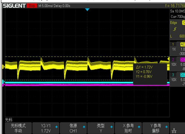
图(5) 25% ~ 50%负载动态波形 (28V)
