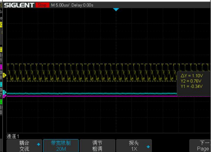
图(4) 电源关机波形 (28V)
