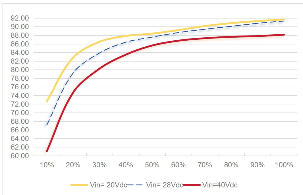
图 6.2 效率曲线图
