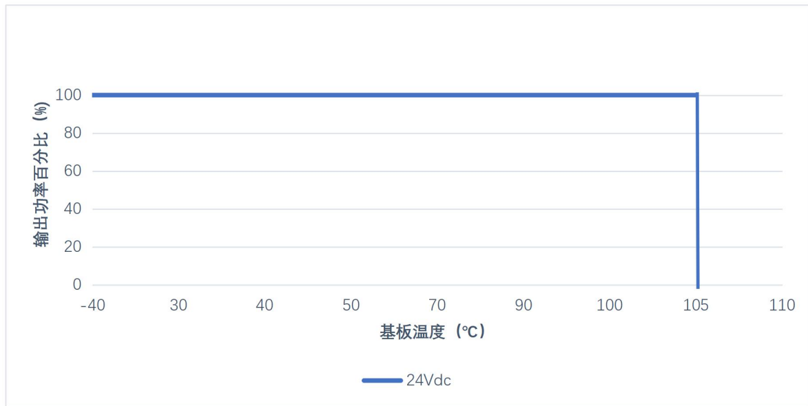
图 6.1 降额曲线图
