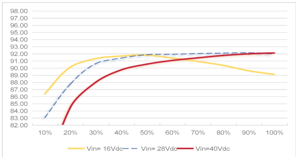
图 6.2 效率曲线
