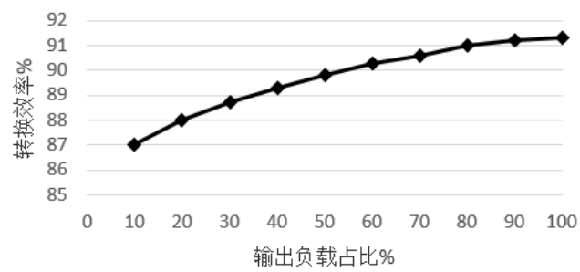
48V 输入负载效率曲线
