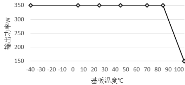
24V 输入降额曲线
