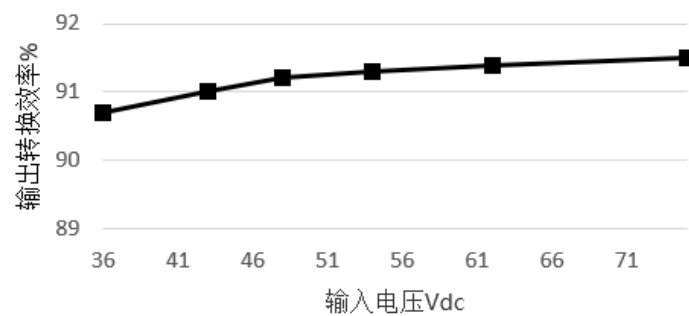
满载输出输入效率曲线
