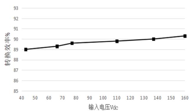
满载输出输入效率曲线
