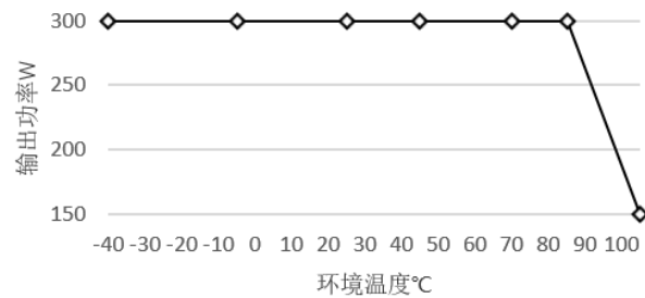
110V 输入降额曲线
