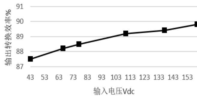
满载输出输入效率曲线
