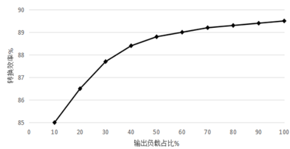
满载输出输入效率曲线
